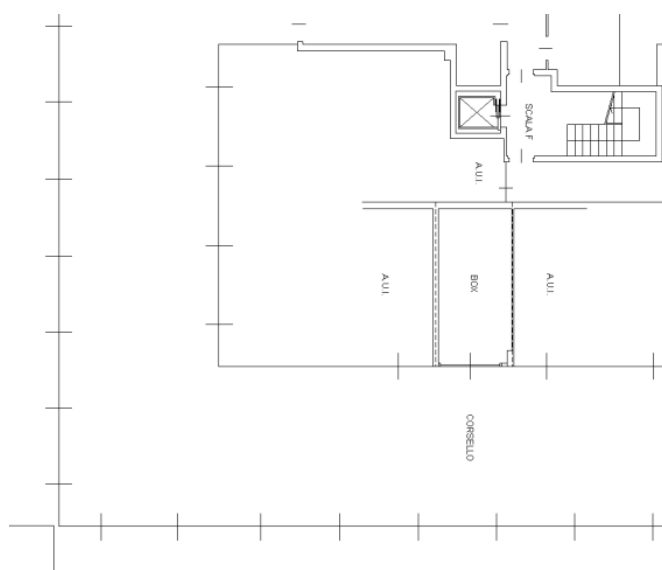
PIANO INTERRATO (vano autorimessa)
